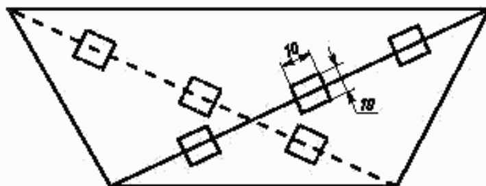
Рисунок Б.2 — Схема расположения квадратов на макрошлифе
