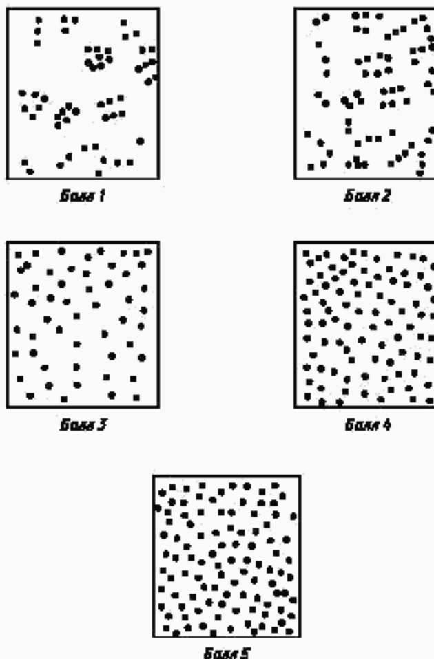
Рисунок Б.1 — Шкала пористости алюминиевых сплавов
