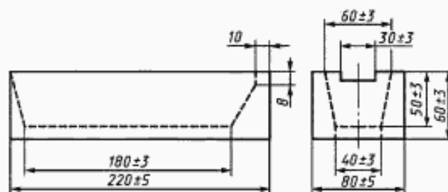
Рисунок 1 — Изложница
