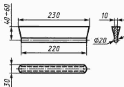
Рисунок 4 — Заготовка для вырезки образцов
