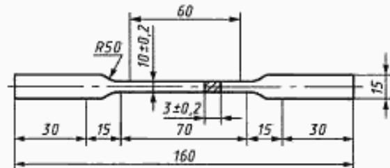
Рисунок 3 — Форма и размеры образца при литье под давлением
